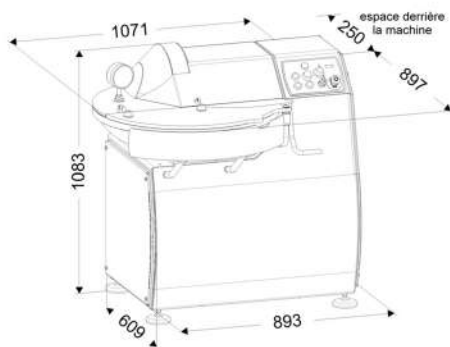
Rozměry Titane 40-2 & 45V
